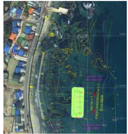
계획 평면도
